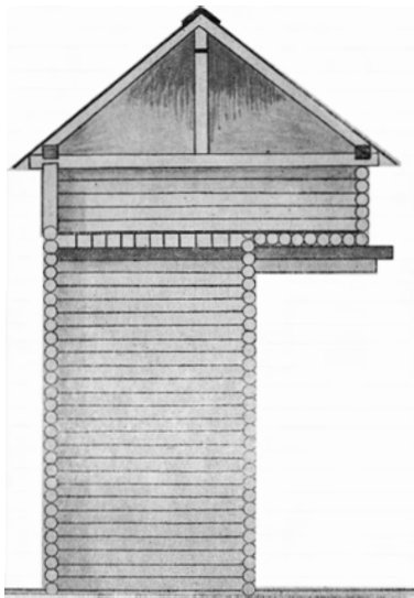
Разрез стены (составной). Реконструкция. (Воронежский край на южных рубежах России (XVII–XVIII вв.) Воронеж, 1981).
