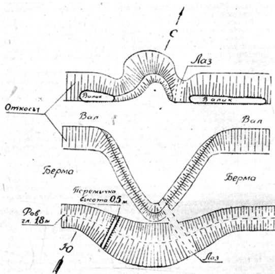
Козловский вал. XVII в. План городка № 5.
