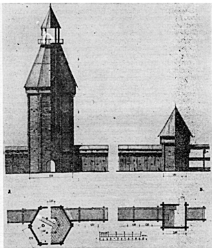
Деревянные башни крепости Острогожска. Московская дозорная; рядовая глухая.
