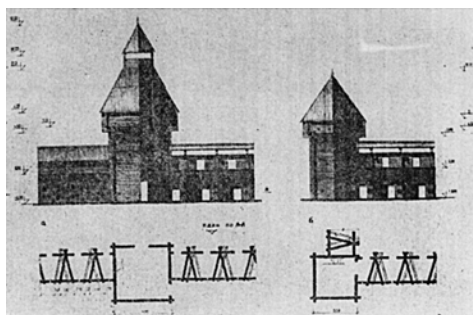
Деревянные башни крепости Коротоаяка. Московская проезжая; угловая глухая.
