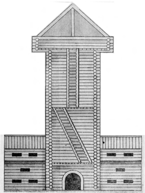
Большая башня. Реконструкция. (Воронежский край на южных рубежах России (XVII–XVIII вв.) Воронеж, 1981).
