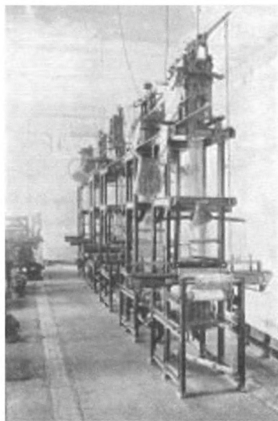
Учебные мастерские Московского прядильно-ткацкого училища на Донской улице. Машины Жаккарда
